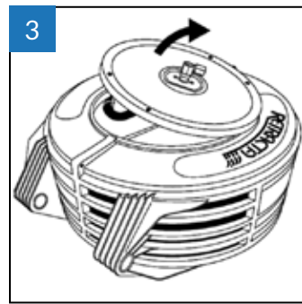
3. Remove sideplate.
